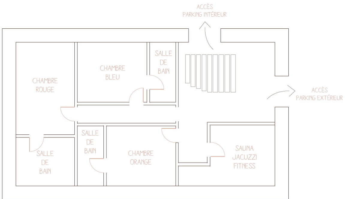
NIVEAU 0
